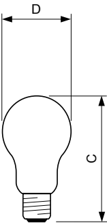
STD 100W E27 230V A60 CL
